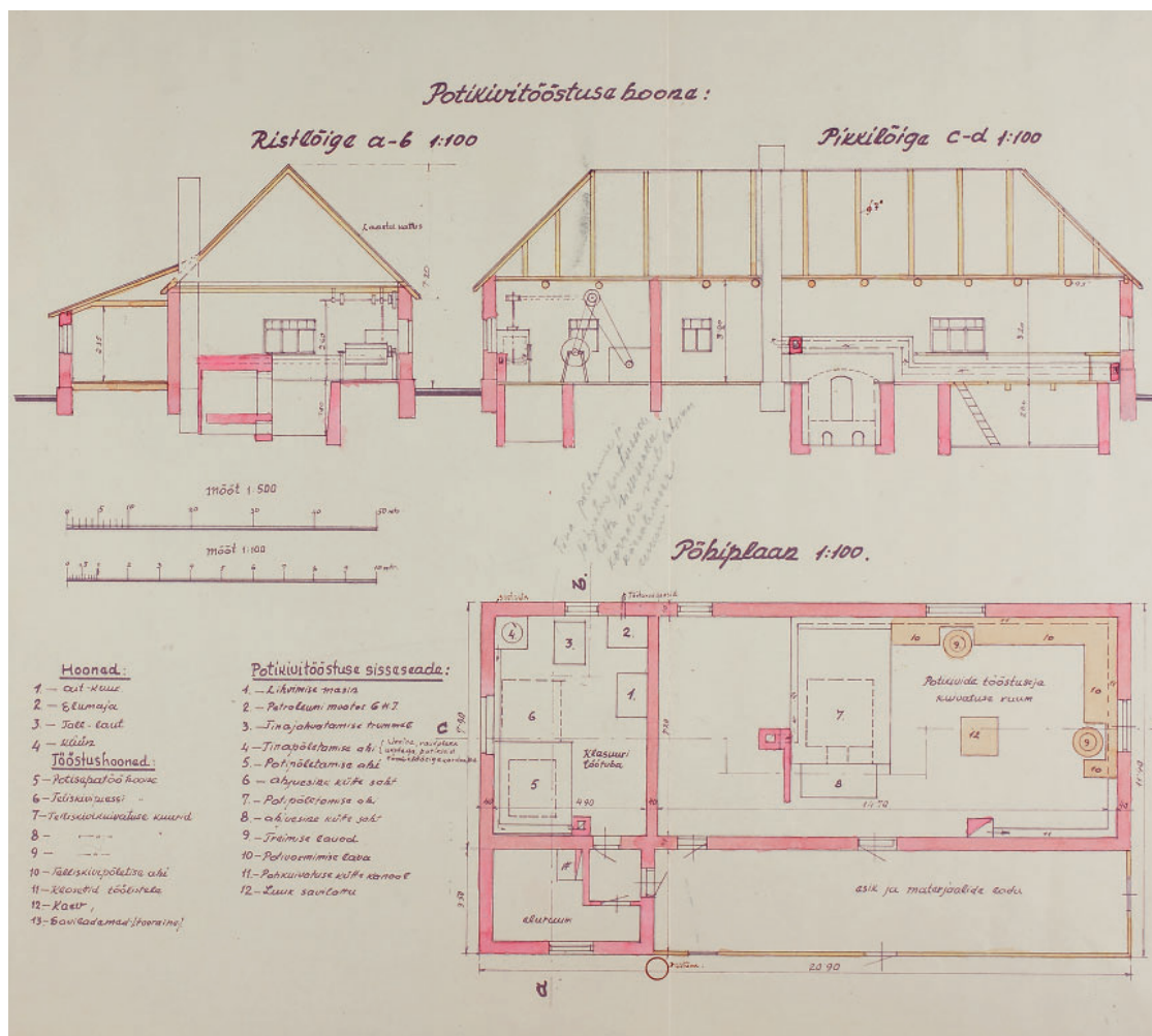
Jn 20. Detail Aleksander Soka savitööstuse plaanist. 1938. ERA.969.4.719.
